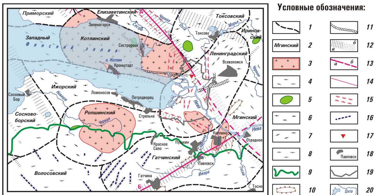
Рис. 6.3. Блоковое строение западной части Ленинградской области согласно, с изменениями и дополнениями. Масштаб 1:1 000 000.
