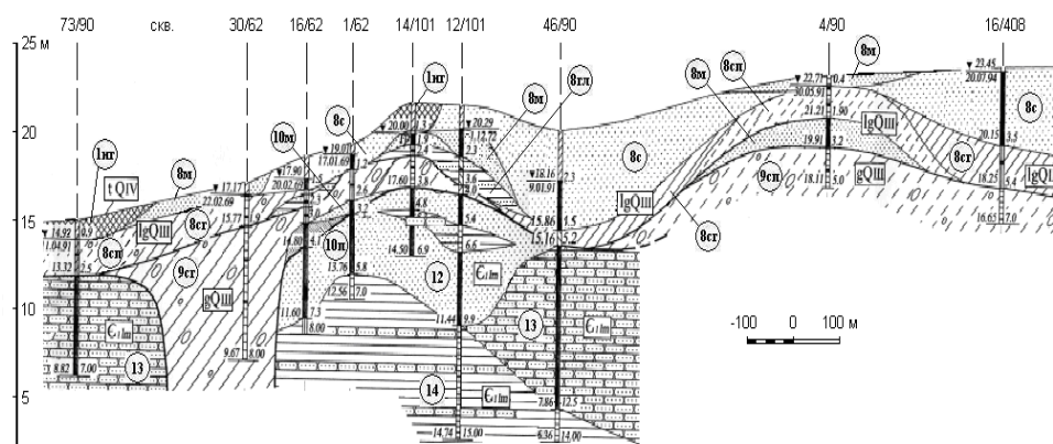
Геологический разрез по линии 1–2
