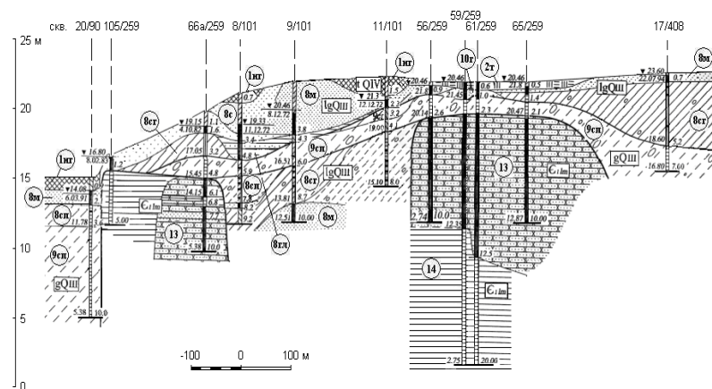
Геологический разрез по линии 1–1
