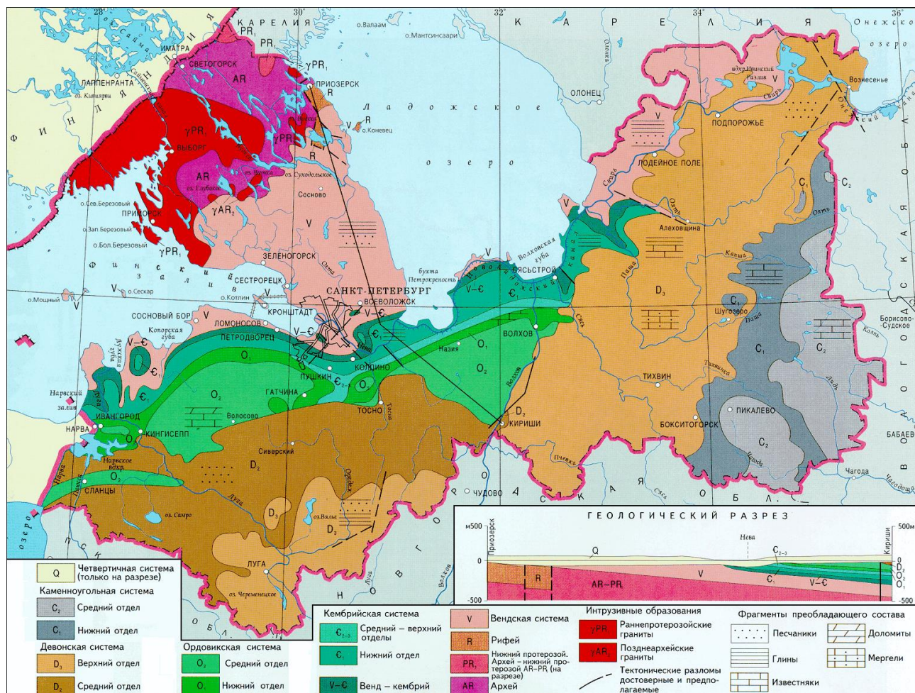
Рис. 6.1. Геологическая карта Ленинградской области, масштаб 1:2 500 000
